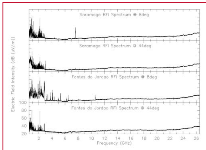
Espectros de RFI medidos en la isla de Santa María (las cuatro gráficas tienen la misma escala vertical)
